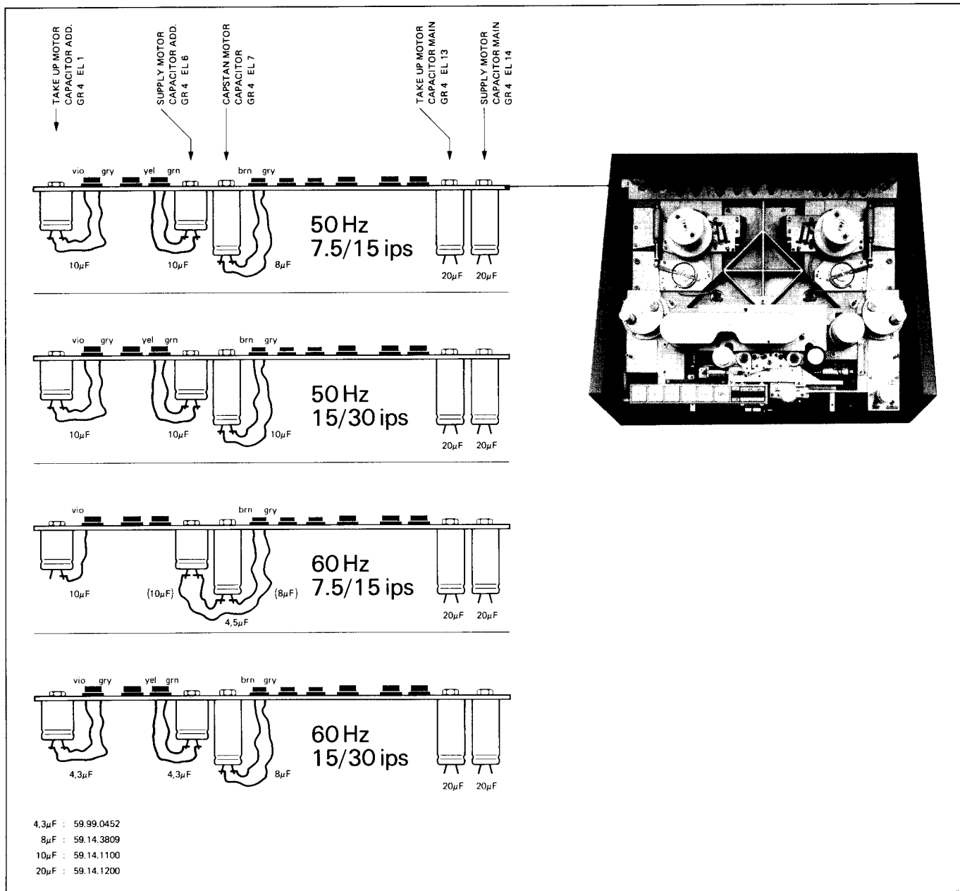
2.2.2 Phasenschieber-Kondensatoren, Übersicht und Werte
